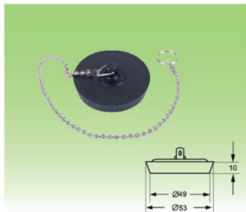
ZDJ 03 Stopper
