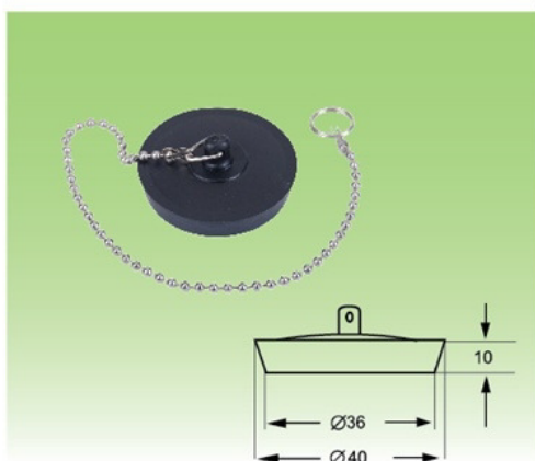
ZDJ 04 Stopper
