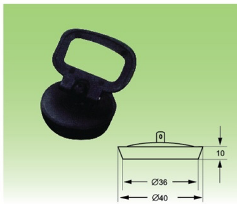
ZDJ 02 Stopper
