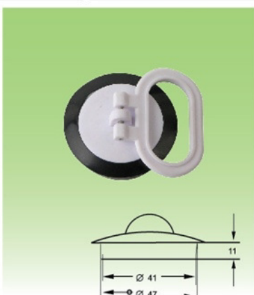
ZDJ 11 Stopper
